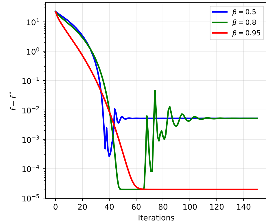
RMSprop: Effect of Decay Parameter
