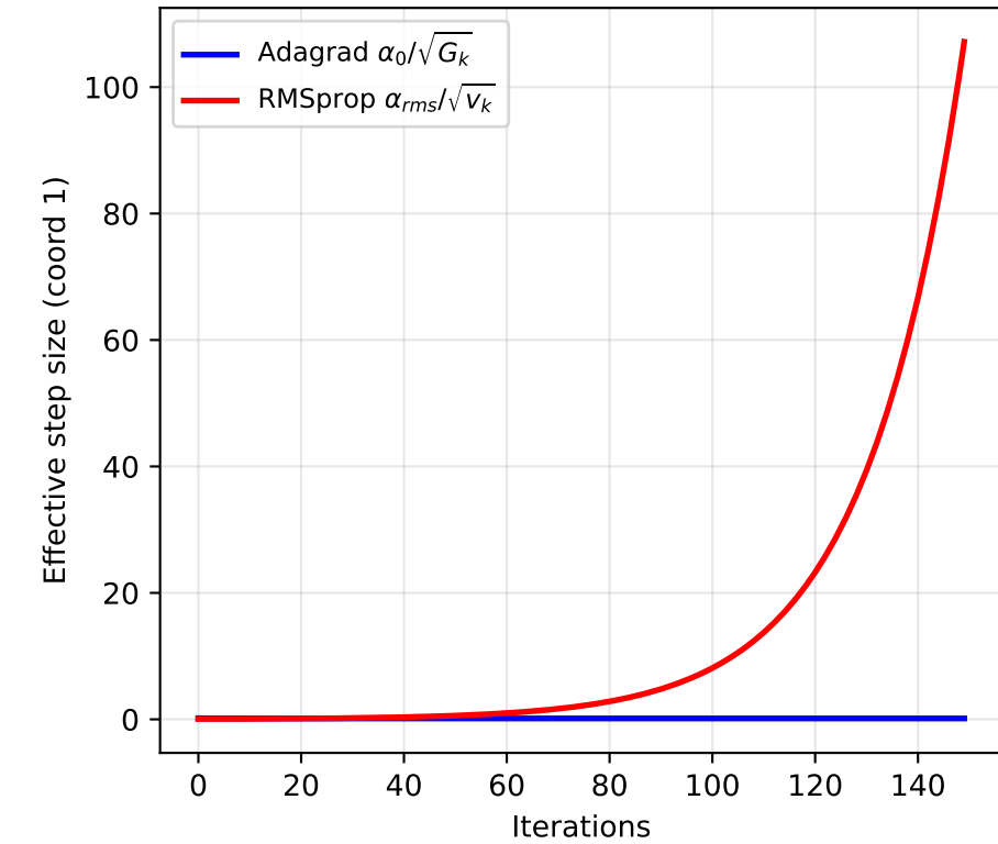
Adagrad vs. RMSprop Step Evolution (same gradient trajectory)
