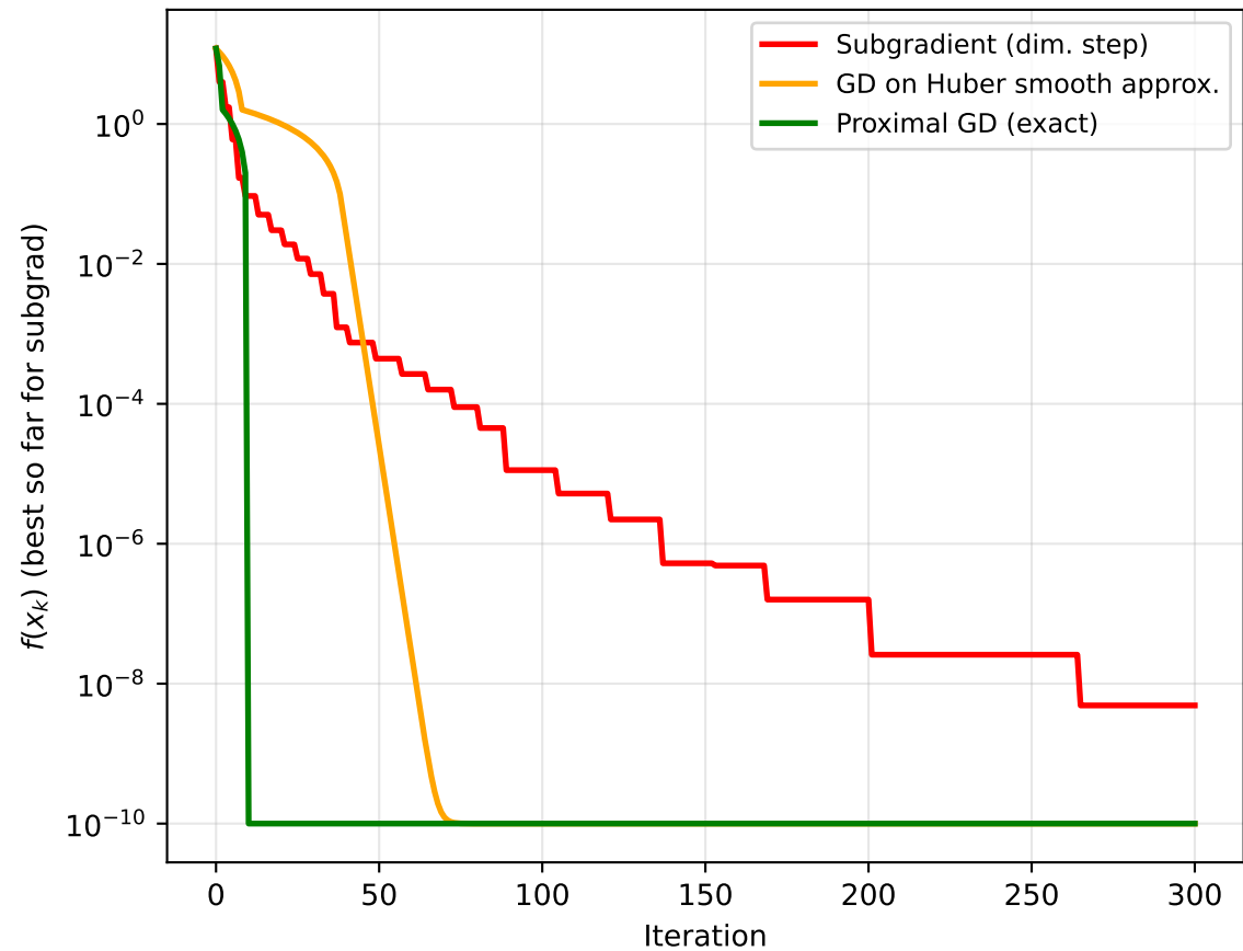
Non-smooth Optimisation: |x_1 - 1| + 5|x_2 - 2|
