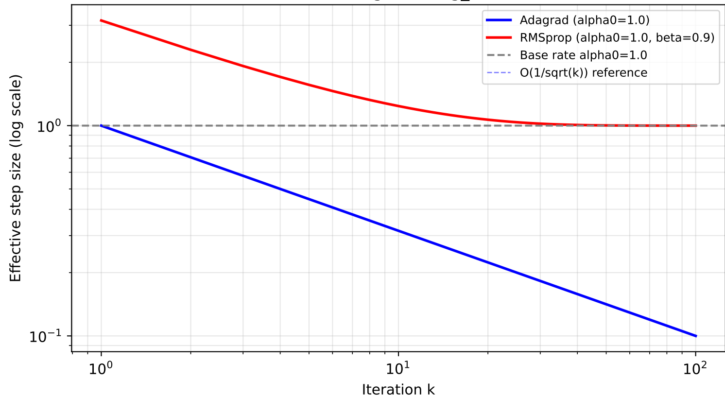
Q1: Adagrad vs RMSprop Effective Step Size Decay (constant gradient g_k=1 )
