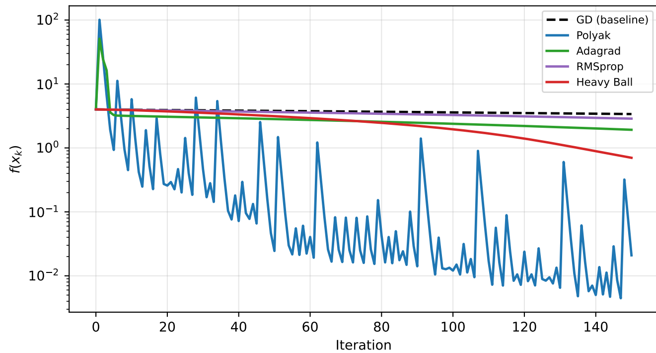
Benchmark C (Rosenbrock) — Q1 Methods
