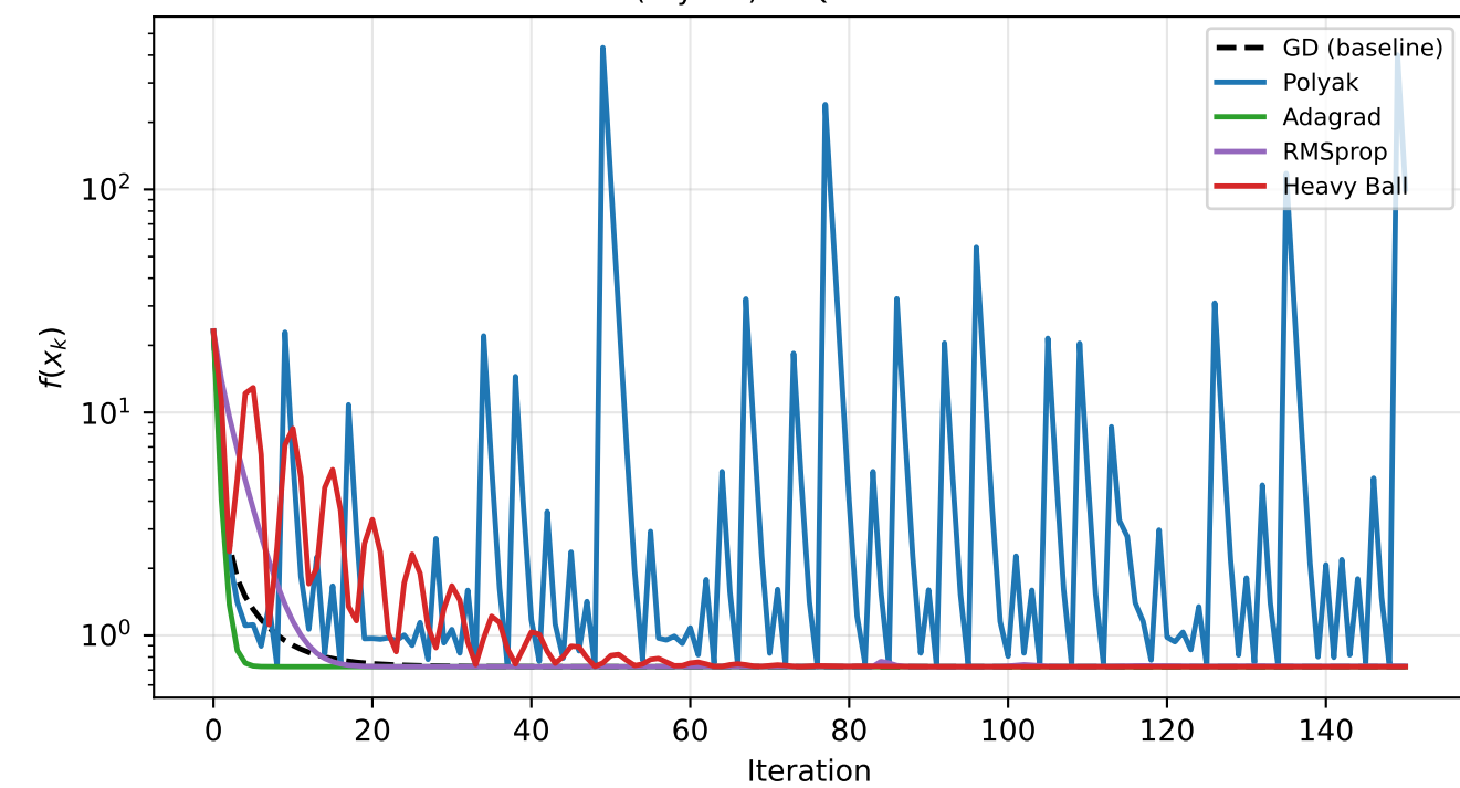
Benchmark C (Rosenbrock) — Q1 Methods
