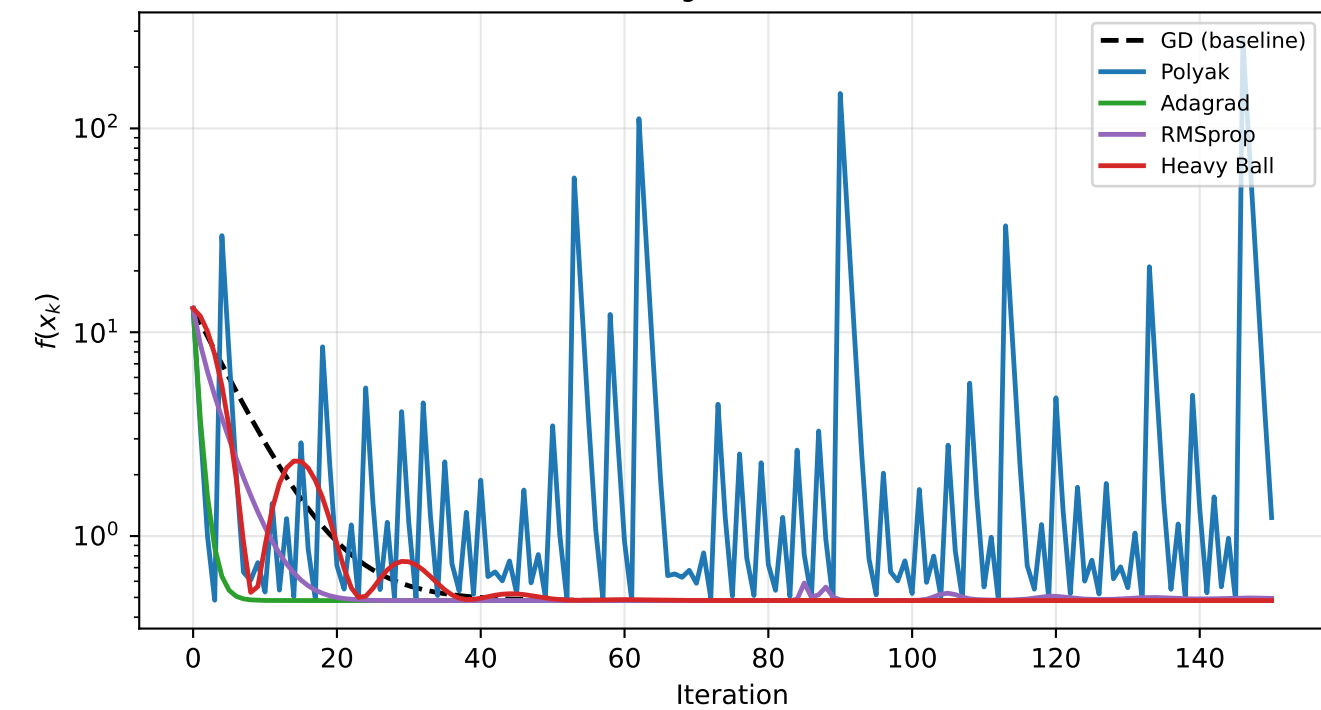
Benchmark B (Toy NN) — Q1 Methods
