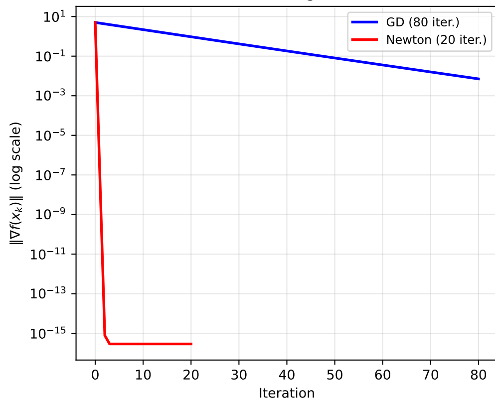
Bench. A: Lin. Reg. ( \kappa \approx 1.12 )
