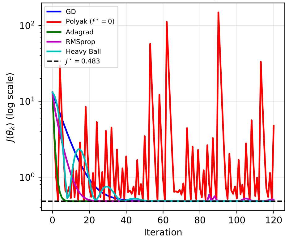
Q1 Bench A: Full Convergence
