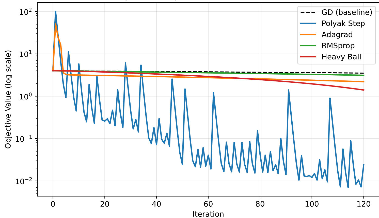
Q1: Convergence Comparison — Benchmark C (Rosenbrock)
