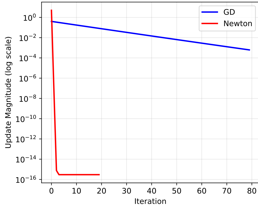
Benchmark A (Linear Reg.)
