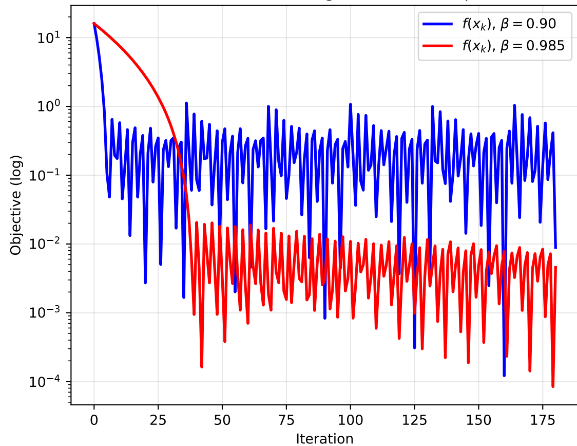
Q6-II: Frank-Wolfe Convergence (Interior Optimum)
