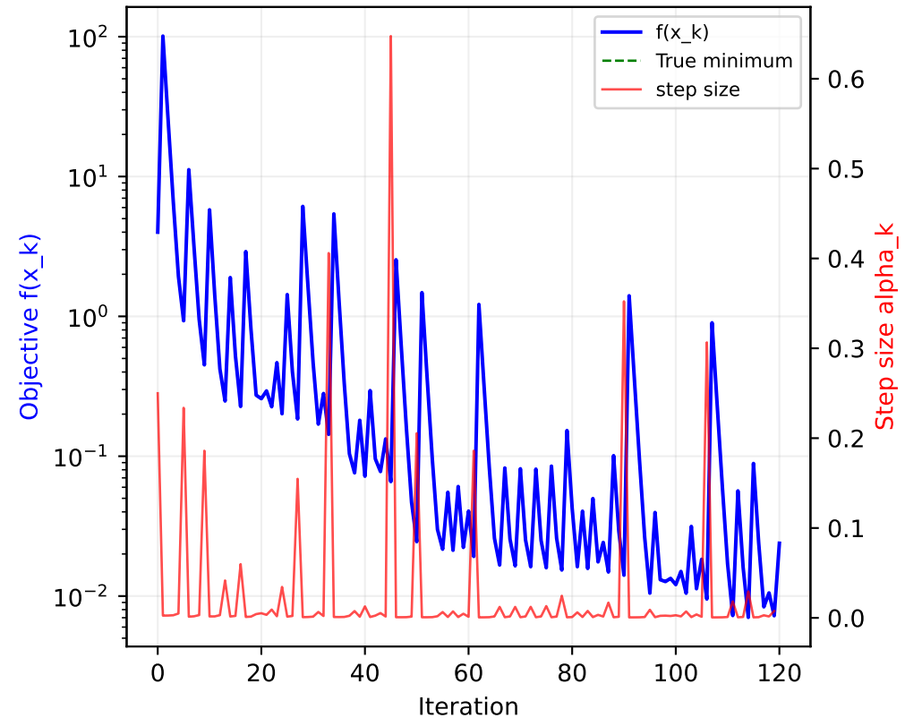
Benchmark C (Rosenbrock) ( f^*=0 exact)
