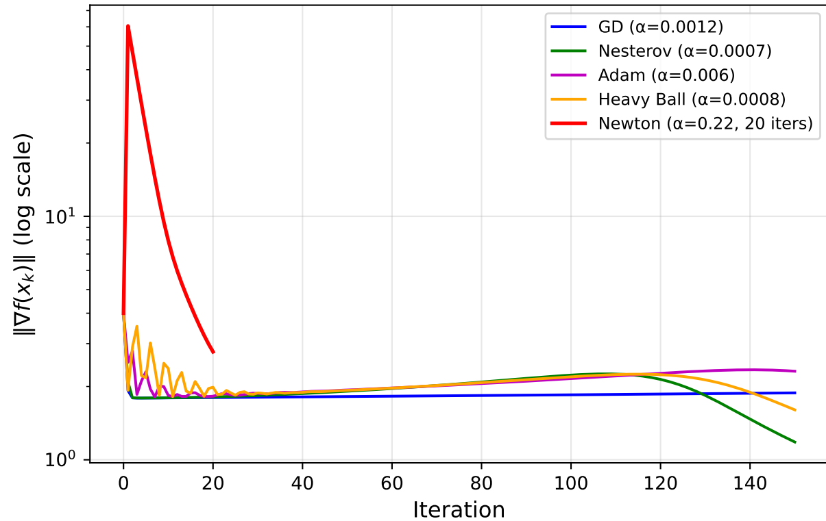
Gradient Norm Decay: Benchmark C (Rosenbrock)
