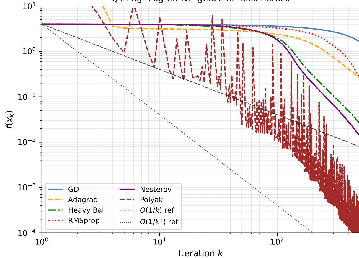
Q1 Log--Log Convergence on Rosenbrock
