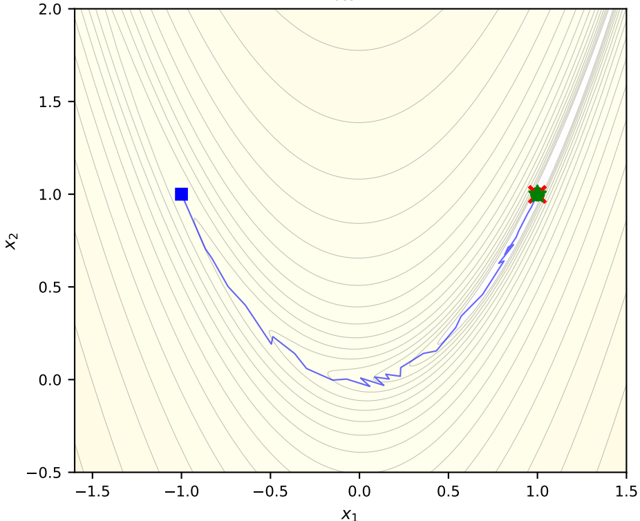
Iter 79: f_{\text{best}} = 0.0000
