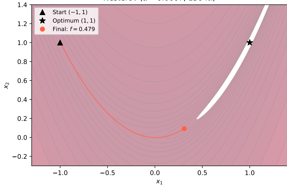
Nesterov ( \alpha = 0.0007 , 150 it.)
