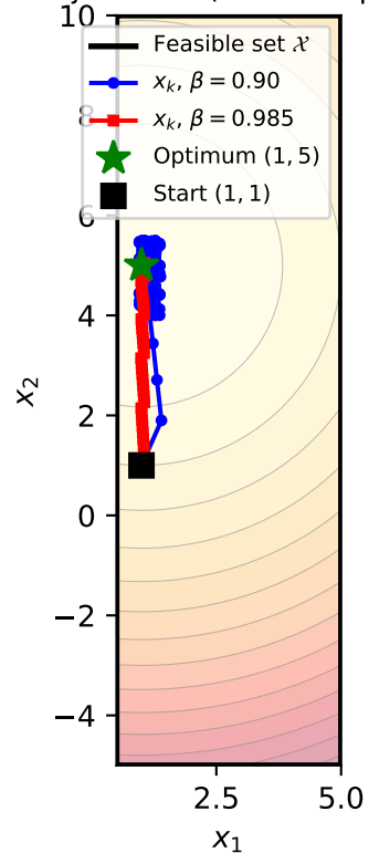
FW Trajectories (Interior Optimum)
