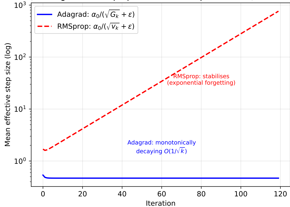
Q1: Adagrad vs RMSprop — Effective Step Evolution (Bench. A)
