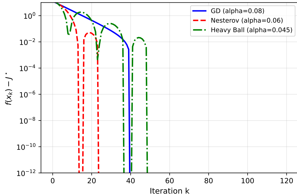
Benchmark A: Actual Suboptimality ( \kappa=1.12 , J^* approx 0.483)
