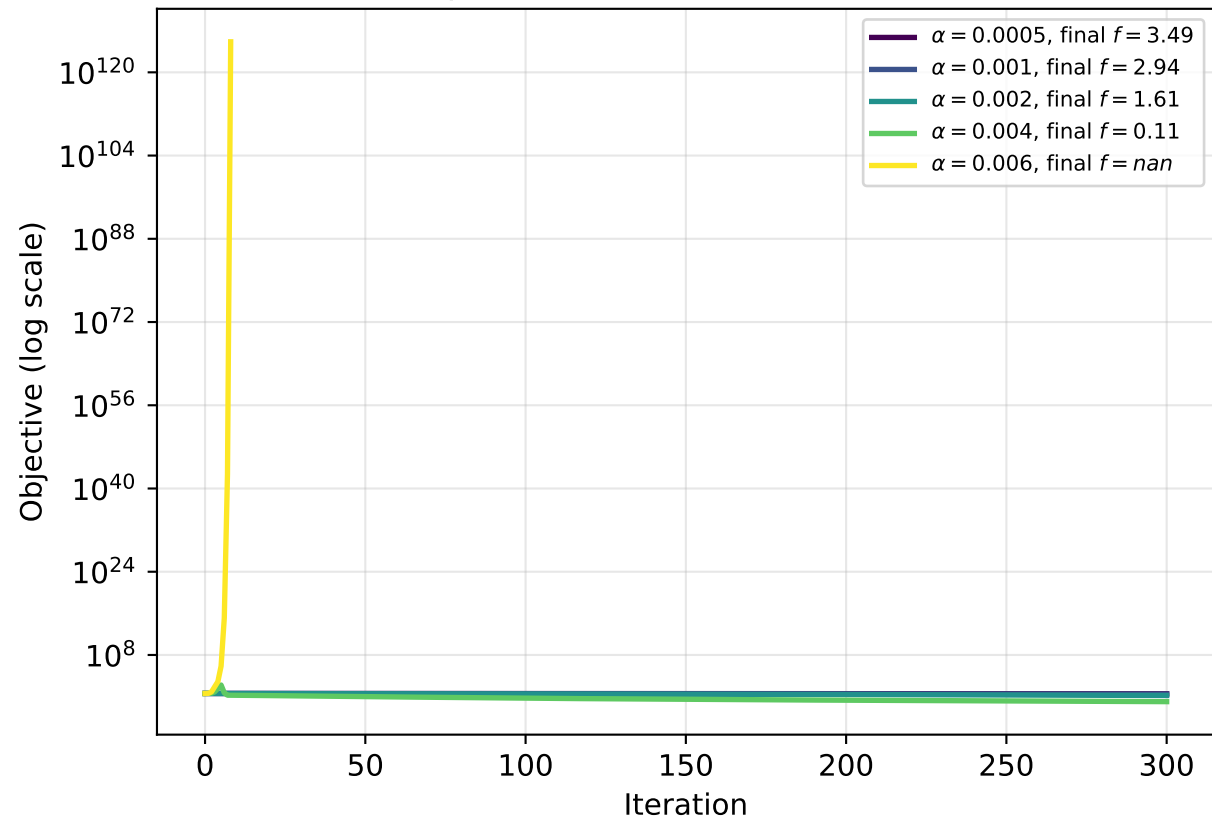
Q1: Effect of Step Size on GD — Benchmark C (Rosenbrock)
