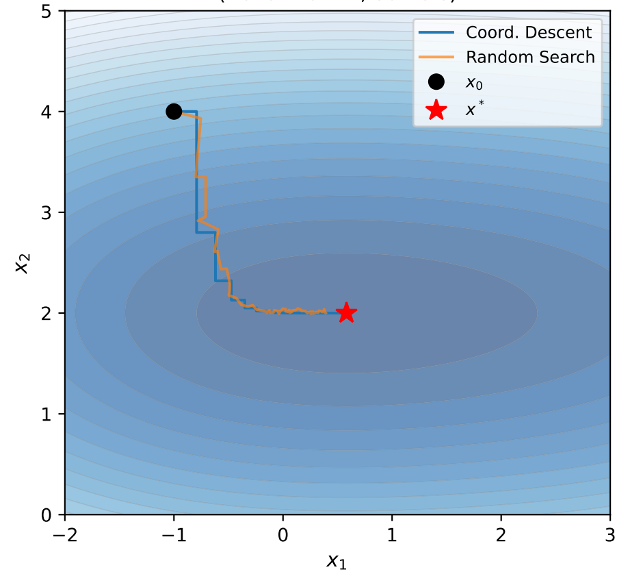
Optimisation Trajectories (Benchmark B, 80 iters)
