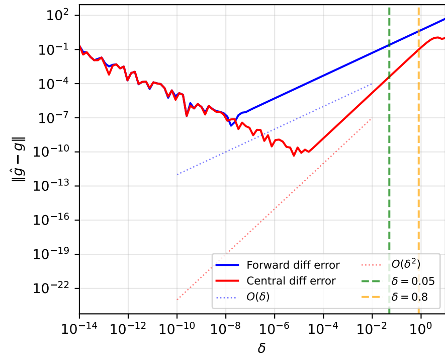
FD vs CD: Gradient Error
