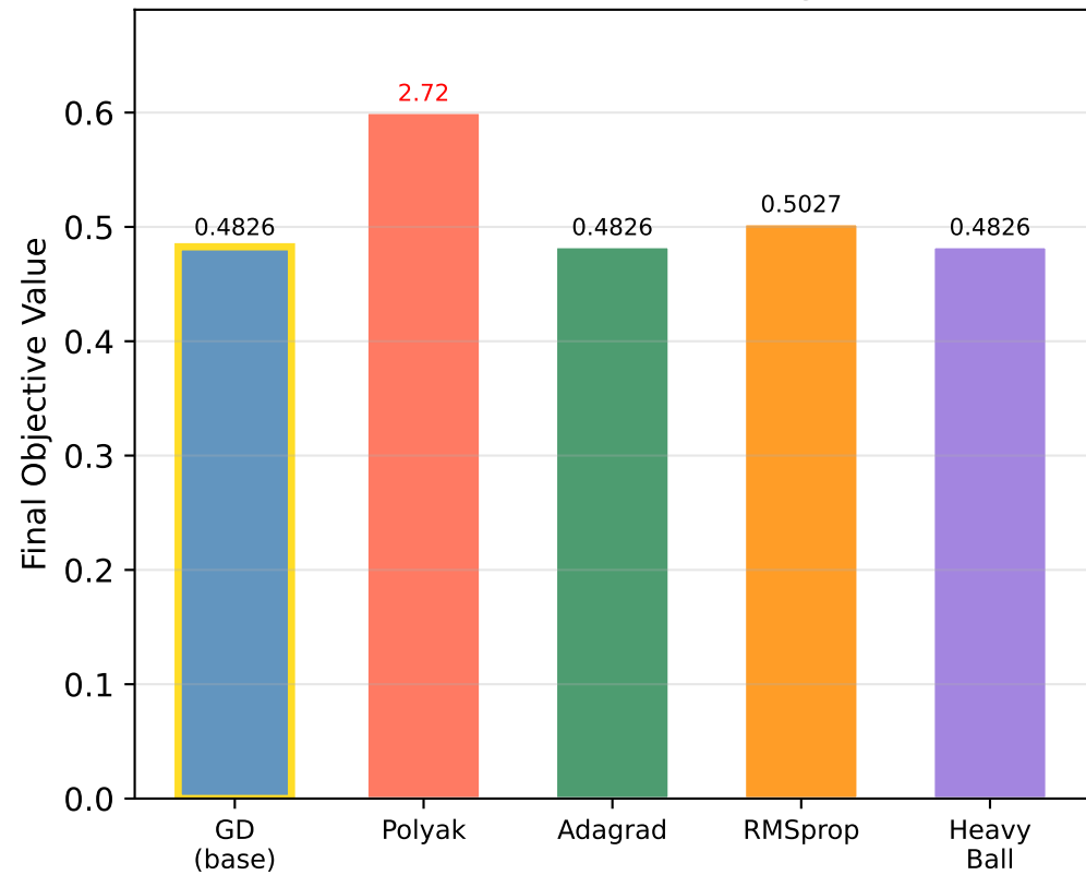
Q1: Benchmark A (Linear Regression)
