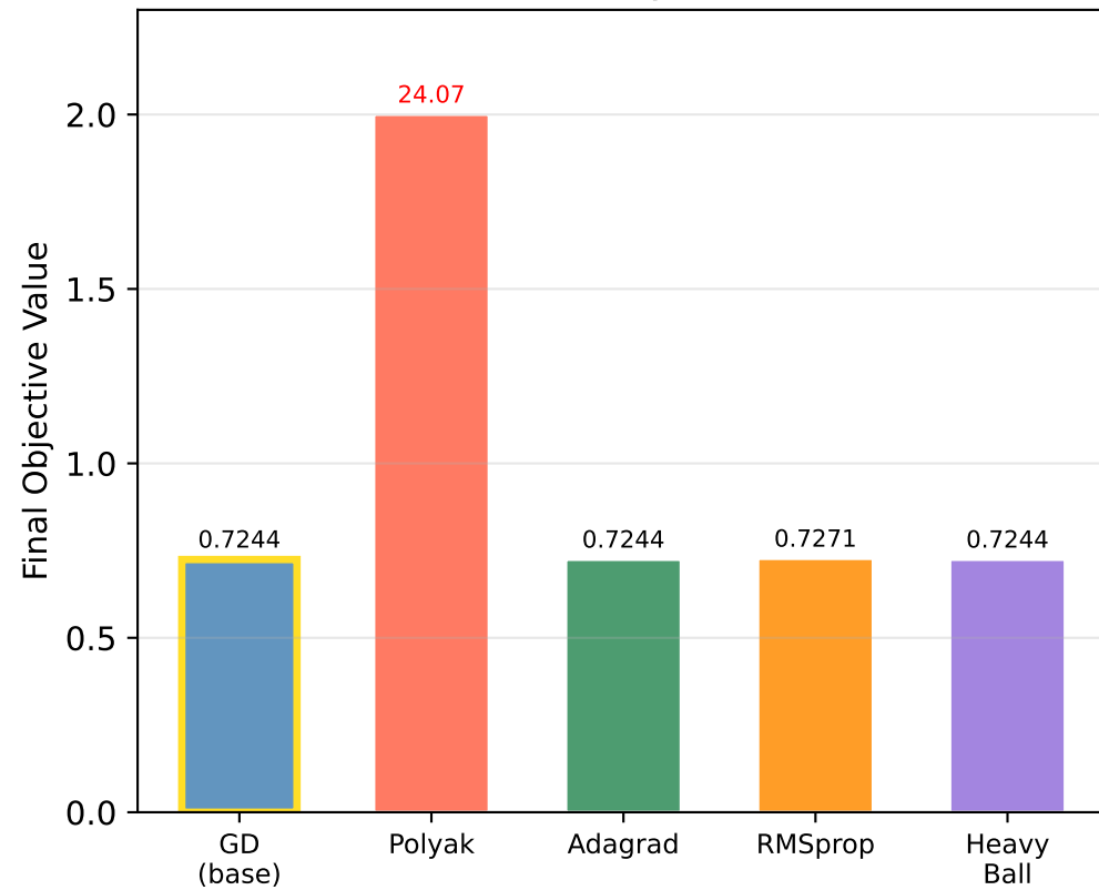
Q1: Benchmark B (Toy Neural Network)
