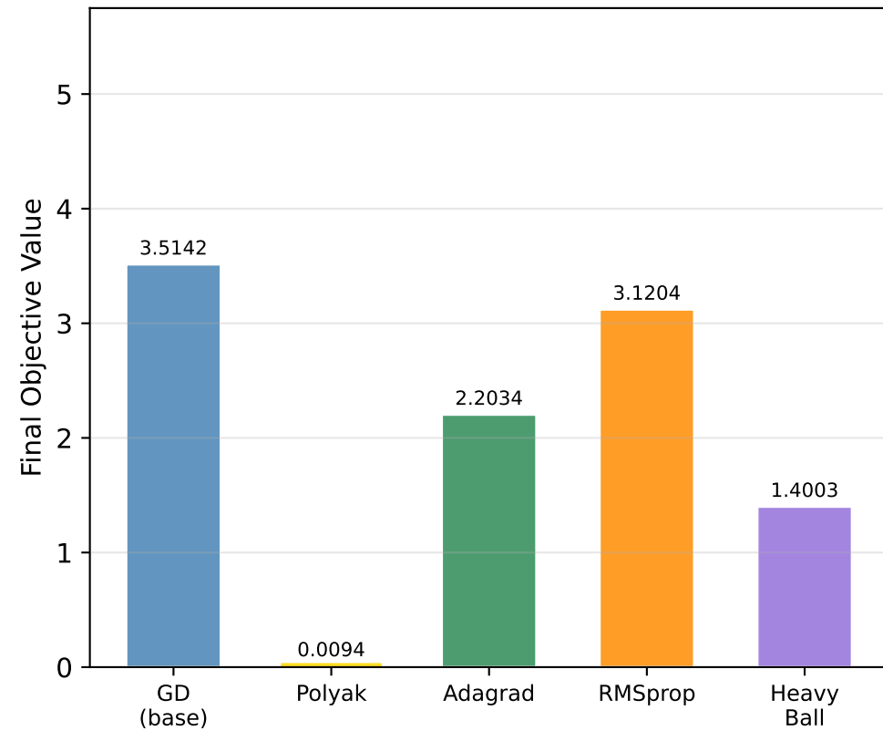
Q1: Benchmark C (Rosenbrock)
