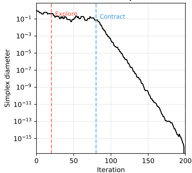
Nelder-Mead Simplex Size
