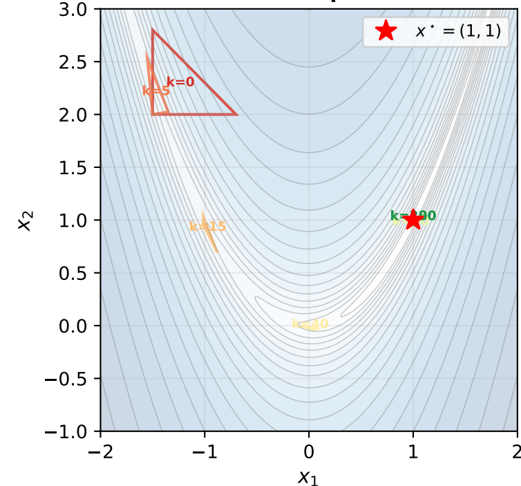
Nelder-Mead Simplex Evolution
