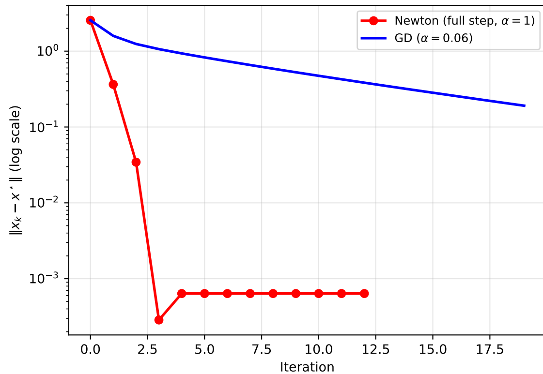
Newton vs GD Error Norm (Benchmark B)
