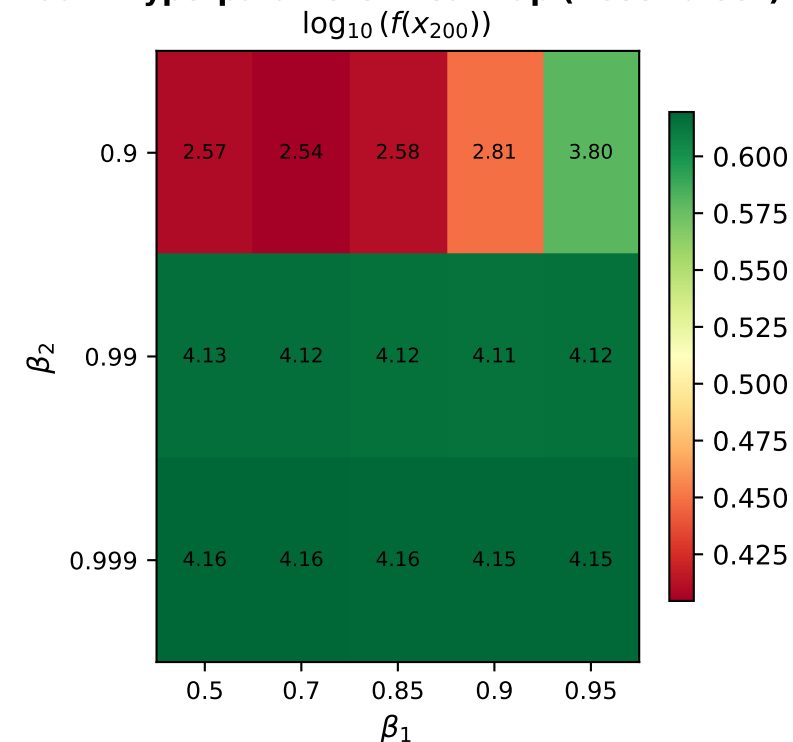
Adam Hyperparameter Heatmap (Rosenbrock)
