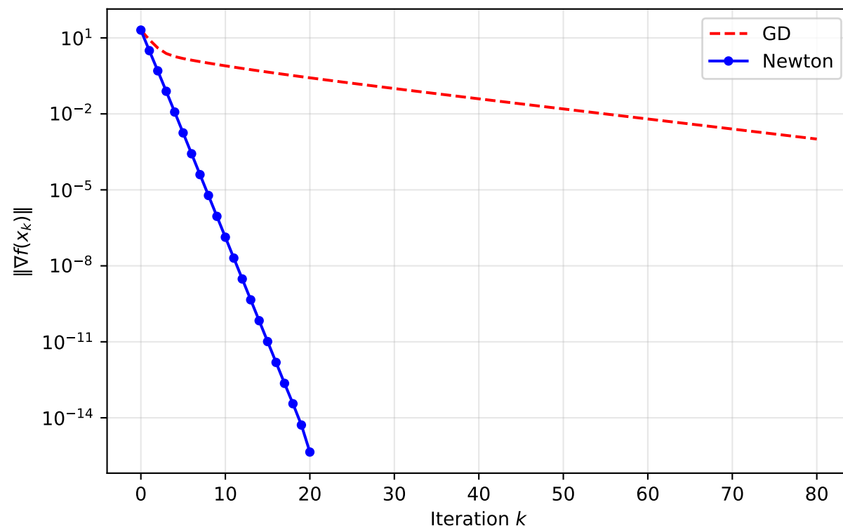
Gradient Norm: Benchmark B
