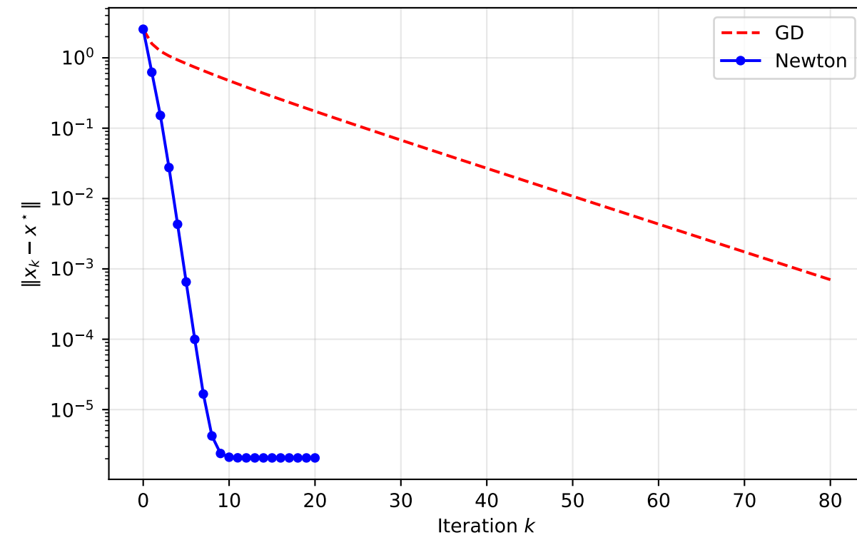
Error Norm: Benchmark B
