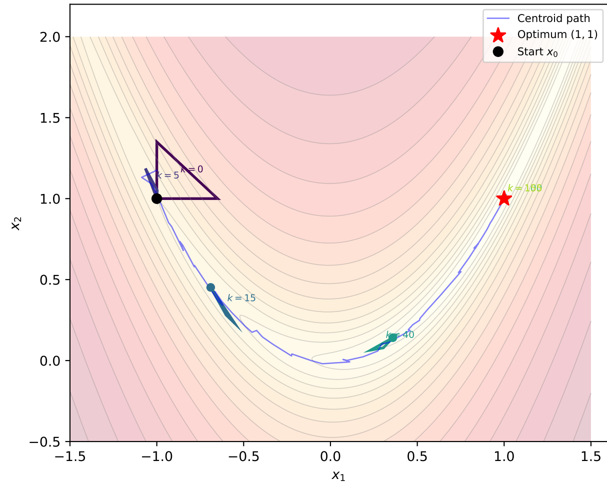
Nelder-Mead Simplex Evolution
