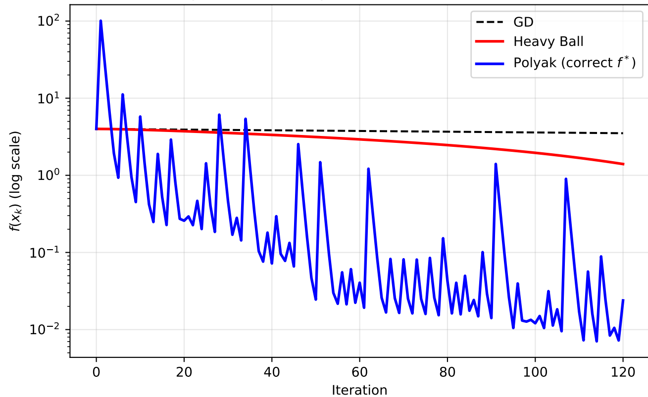
Q1: Convergence Rate Comparison — Benchmark C (Rosenbrock)
