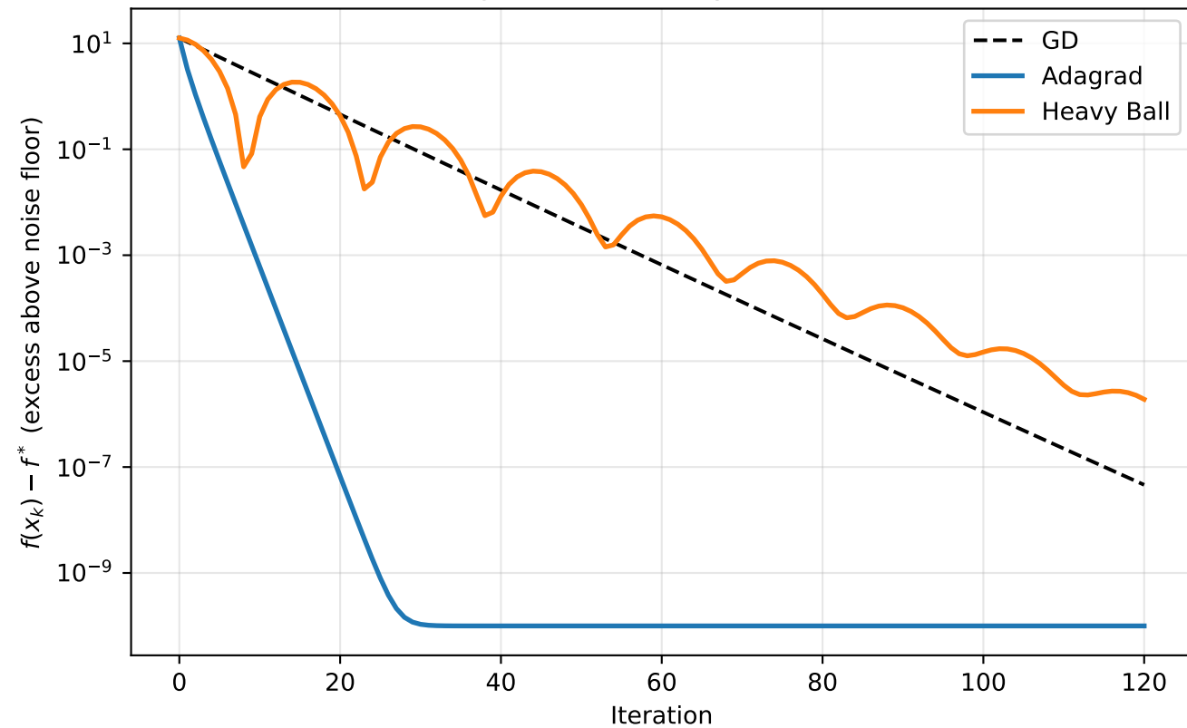
Q1: Convergence Rate Analysis — Benchmark A
