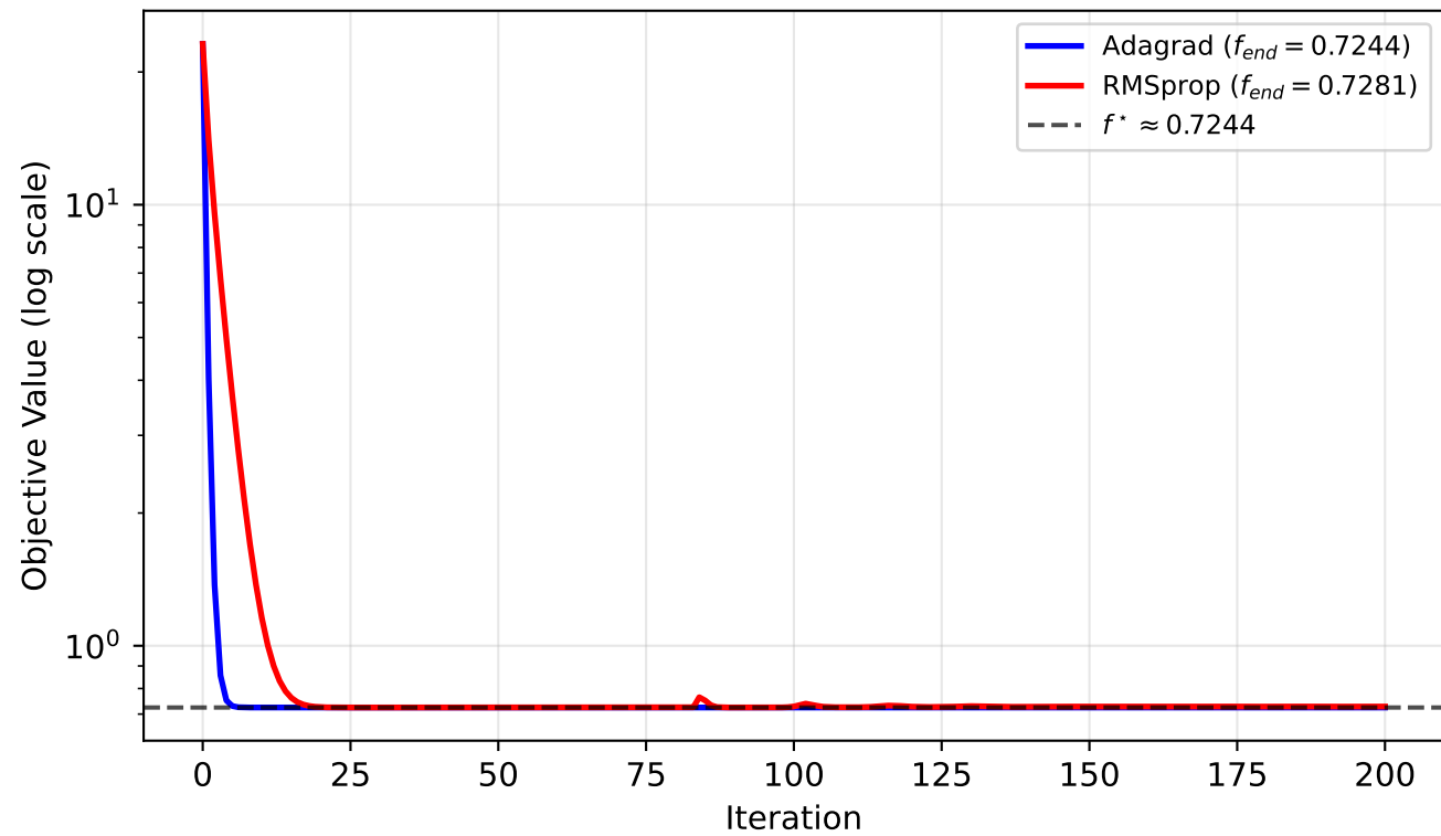
Adagrad vs RMSprop: Convergence (Benchmark B)
