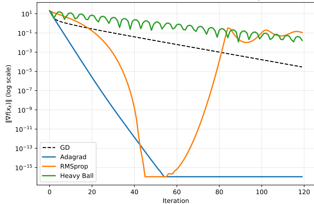
Q1: Gradient Norm Evolution — Benchmark B (Toy NN)
