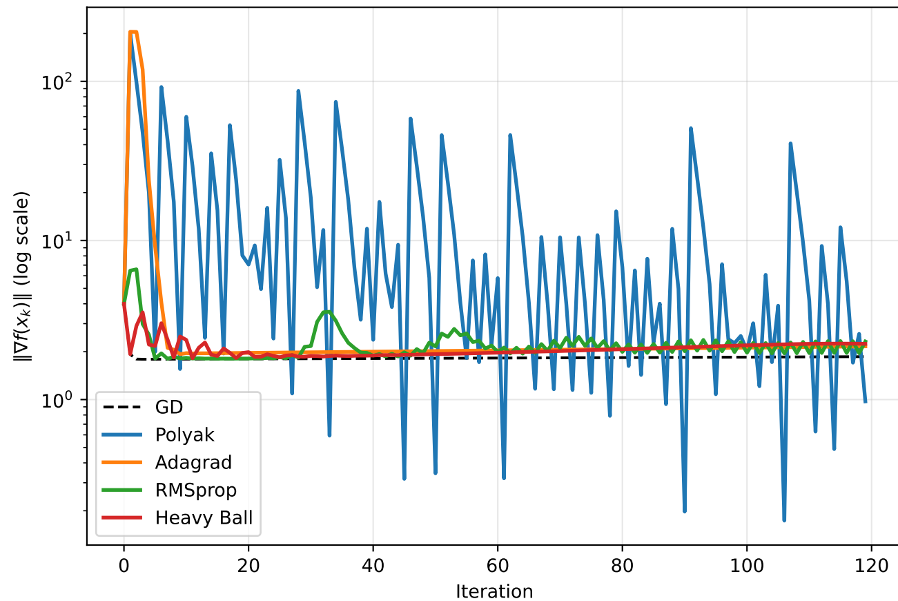
Q1: Gradient Norm Evolution — Rosenbrock
