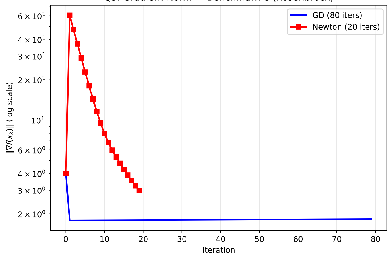
Q3: Gradient Norm — Benchmark C (Rosenbrock)
