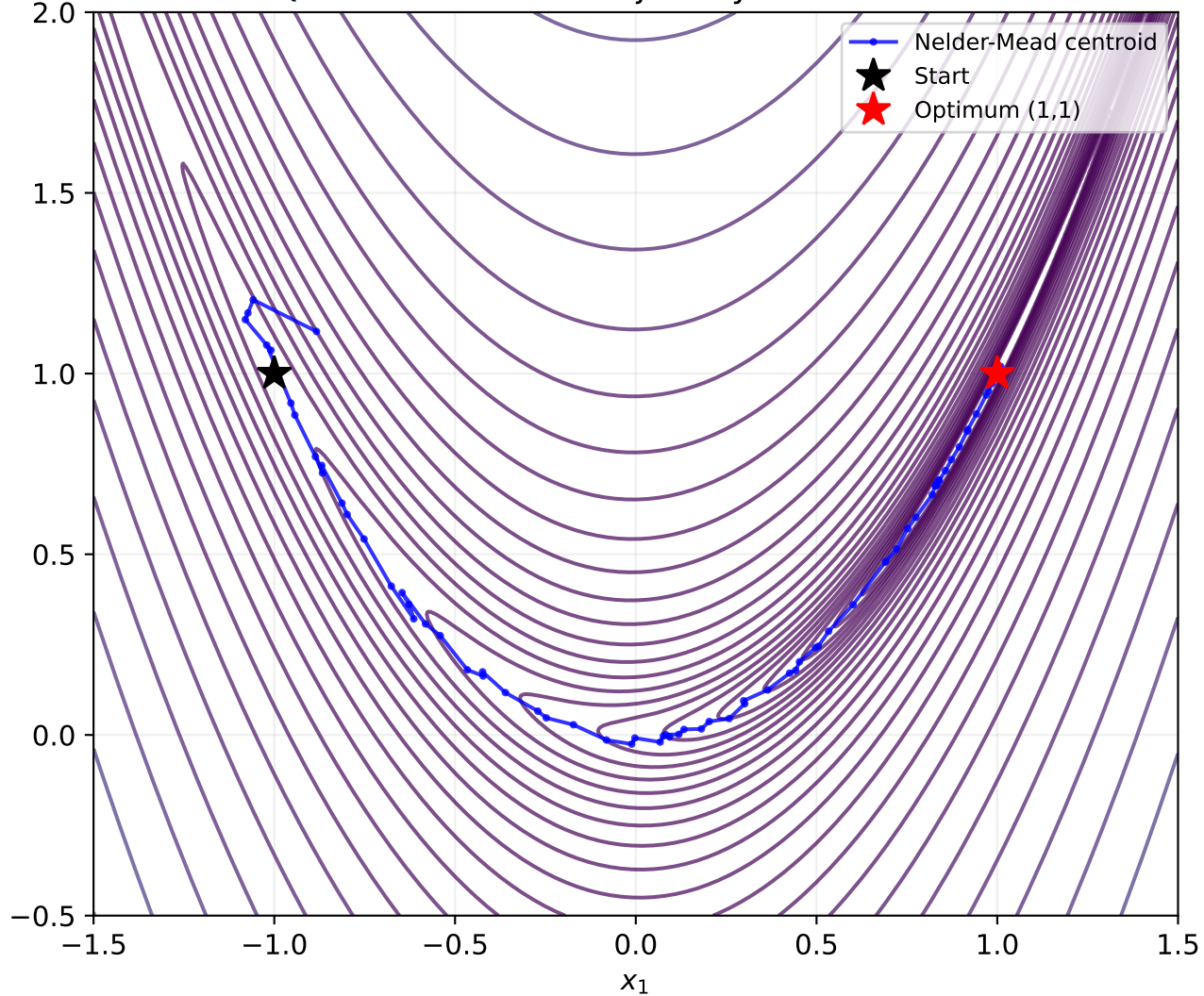
Q4B: Nelder-Mead Trajectory — Rosenbrock
