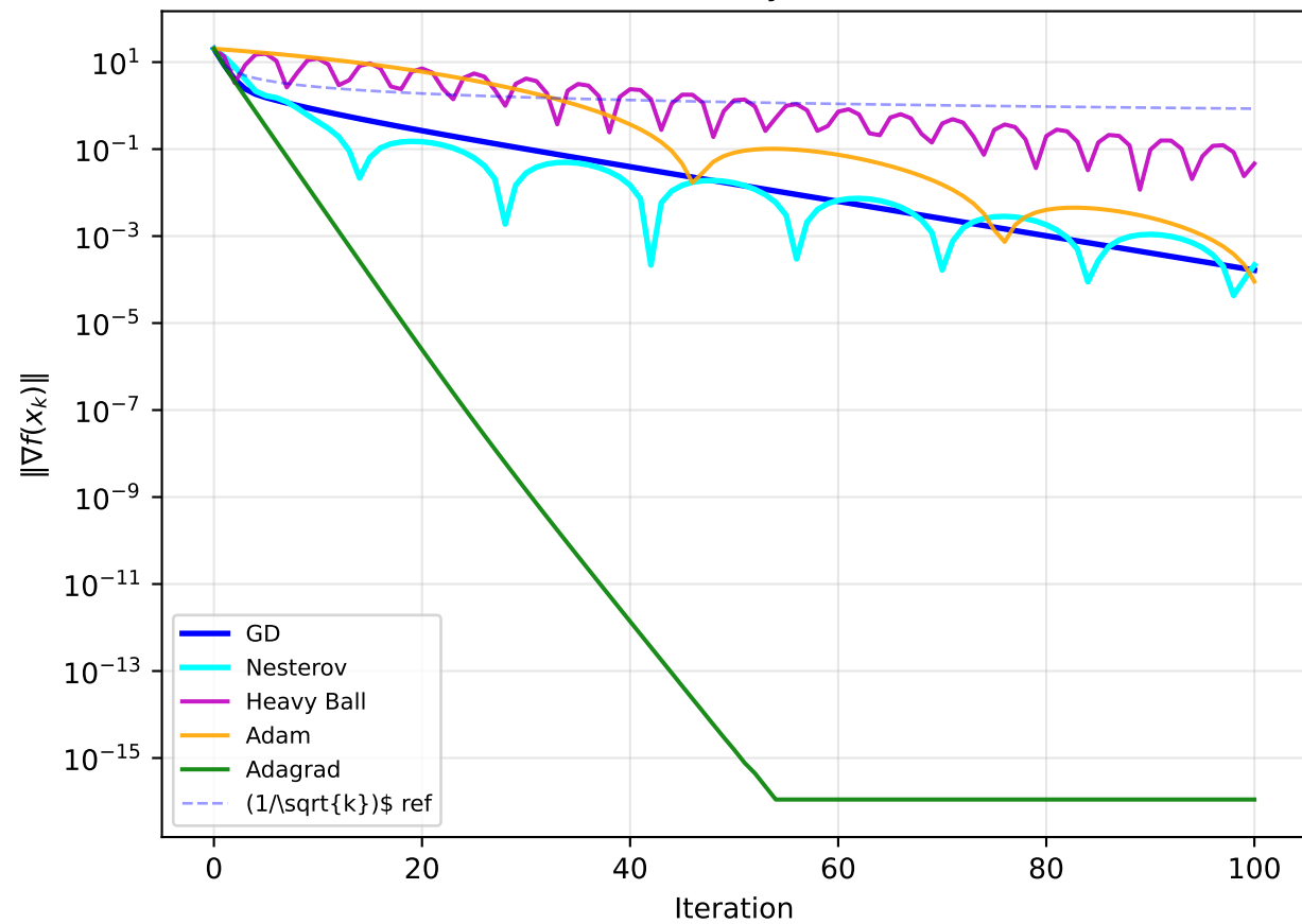
Gradient Norm Decay (Benchmark B)
