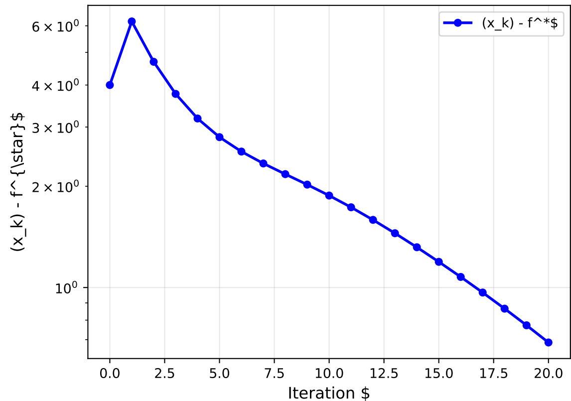
Benchmark C (Rosenbrock)
