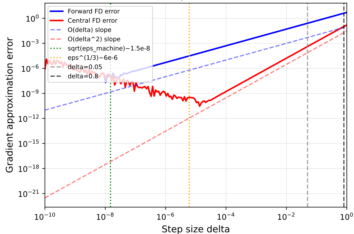
FD Error vs Step Size (Benchmark B)
