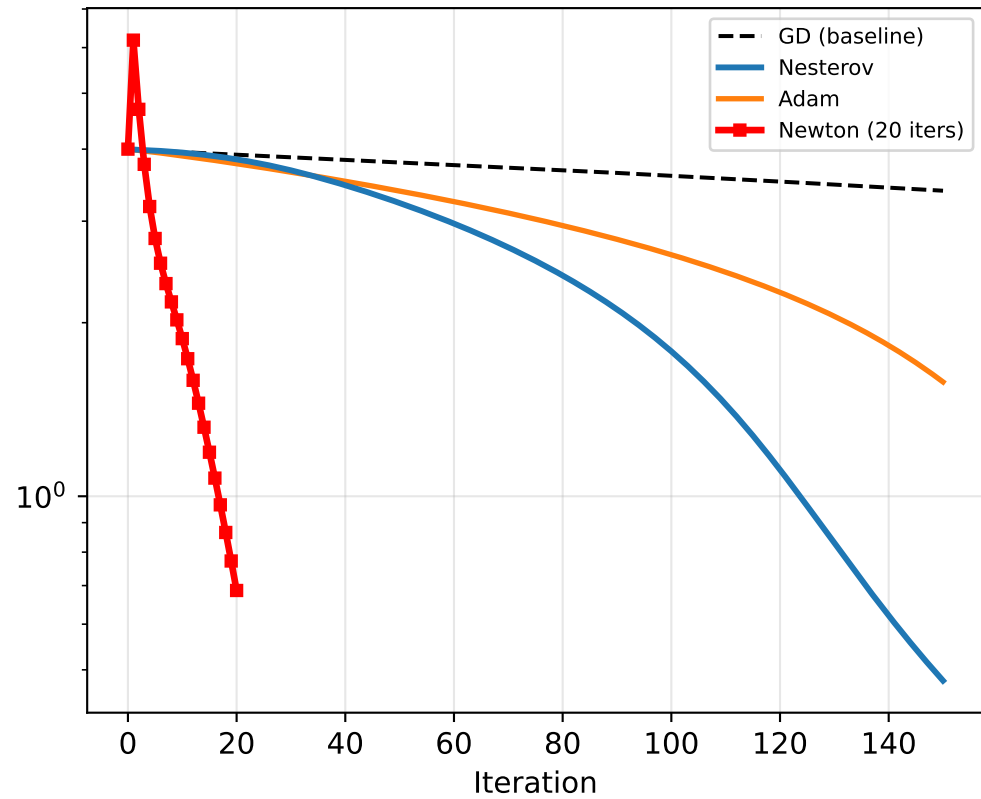
Benchmark C (Rosenbrock)
