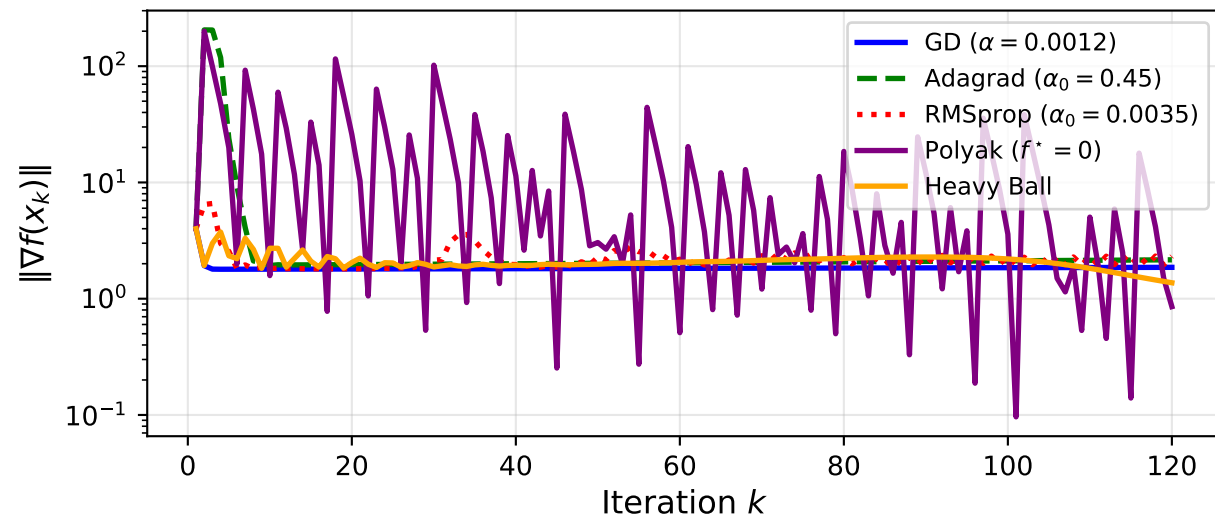
Q1: Gradient Norm vs. Iteration (Benchmark C, Rosenbrock)
