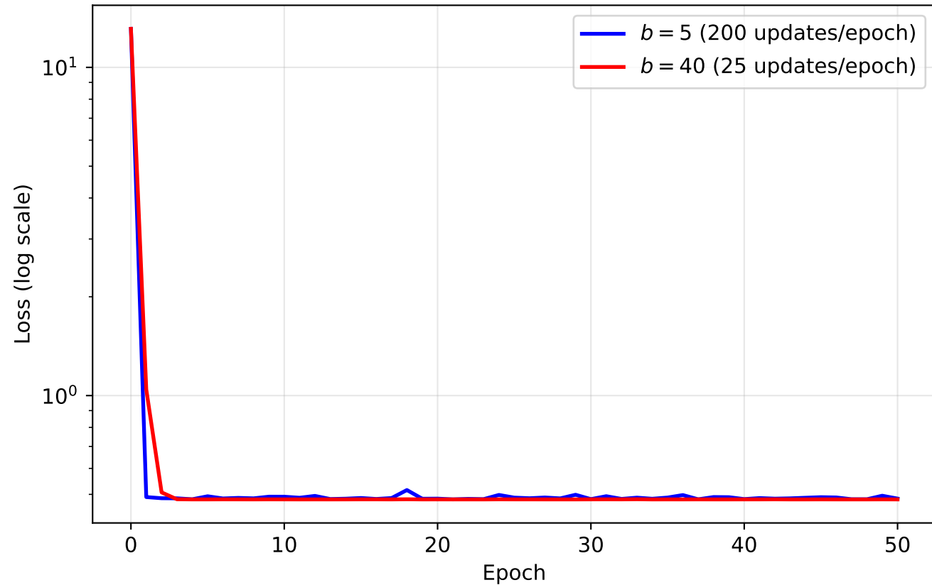
SGD: Loss per Epoch
