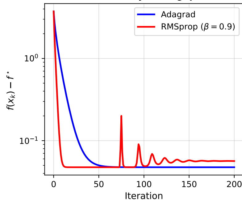
(d) Convergence on Benchmark A (actual objective gap)
