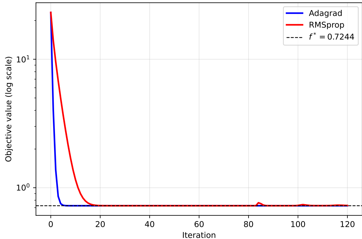
Q1: Adagrad vs RMSprop Convergence — Benchmark B
