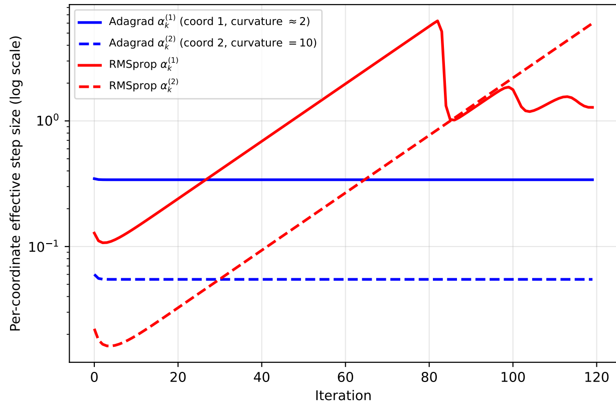
Q1: Per-Coordinate Adaptive Step Sizes — Benchmark B
