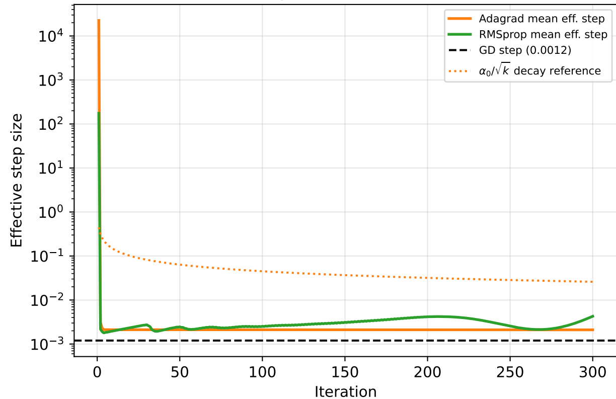
Q1: Effective Step Size Evolution (Benchmark C)
