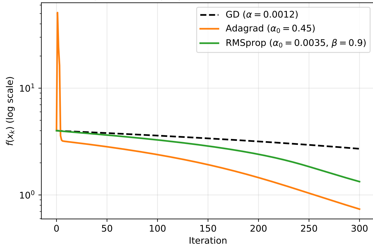
Q1: Adagrad vs RMSprop on Benchmark C (300 iterations)
