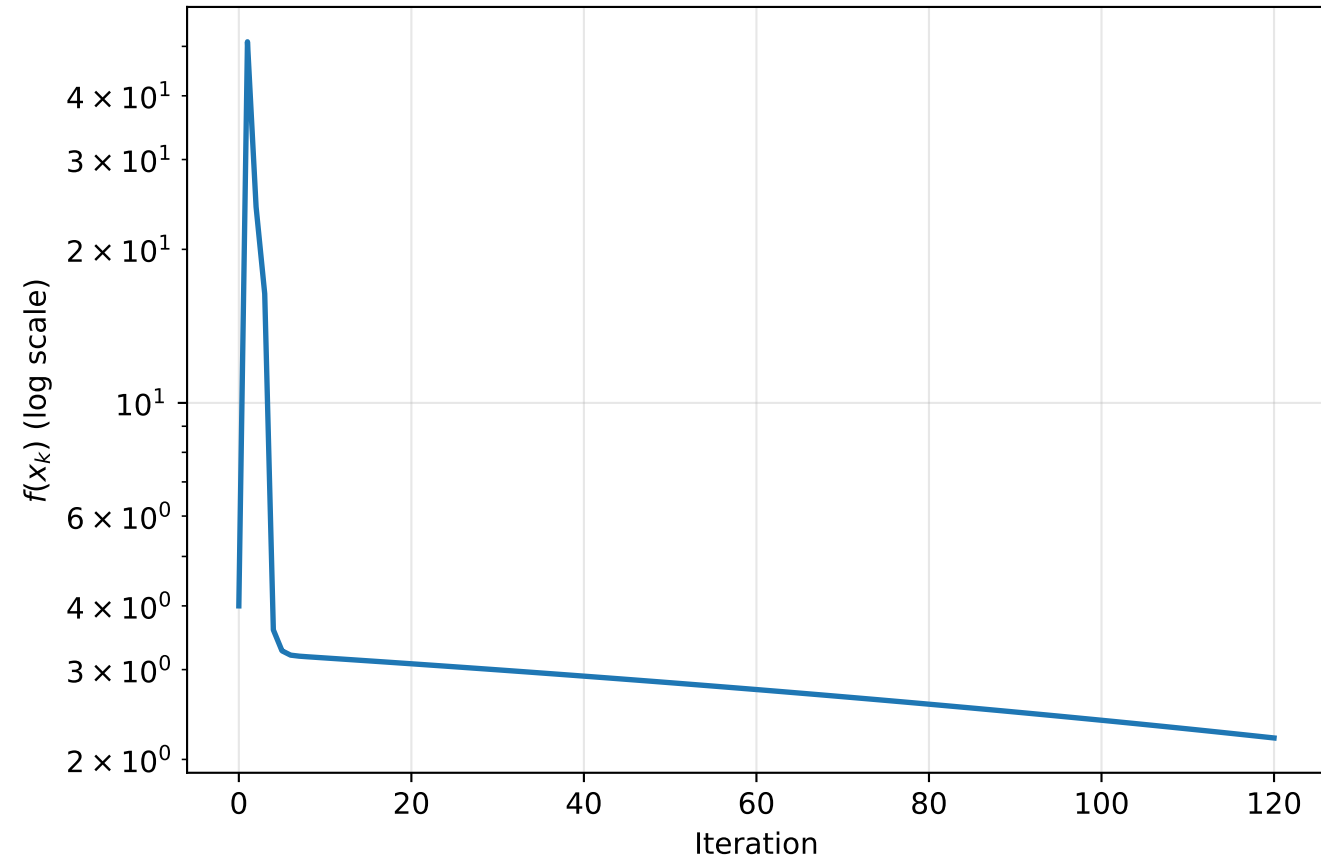
Q1: Adagrad Convergence on Benchmark C
