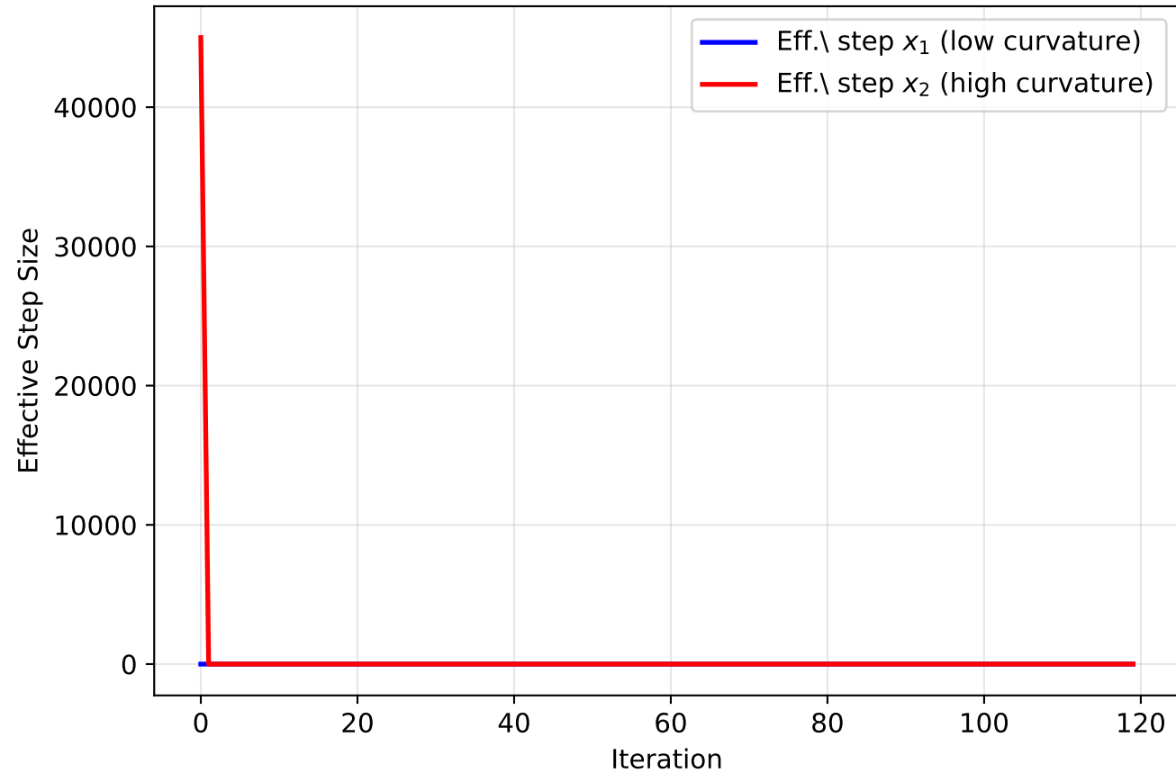
Q1: Adagrad Per-Coordinate Step Size — Benchmark C (Rosenbrock)
