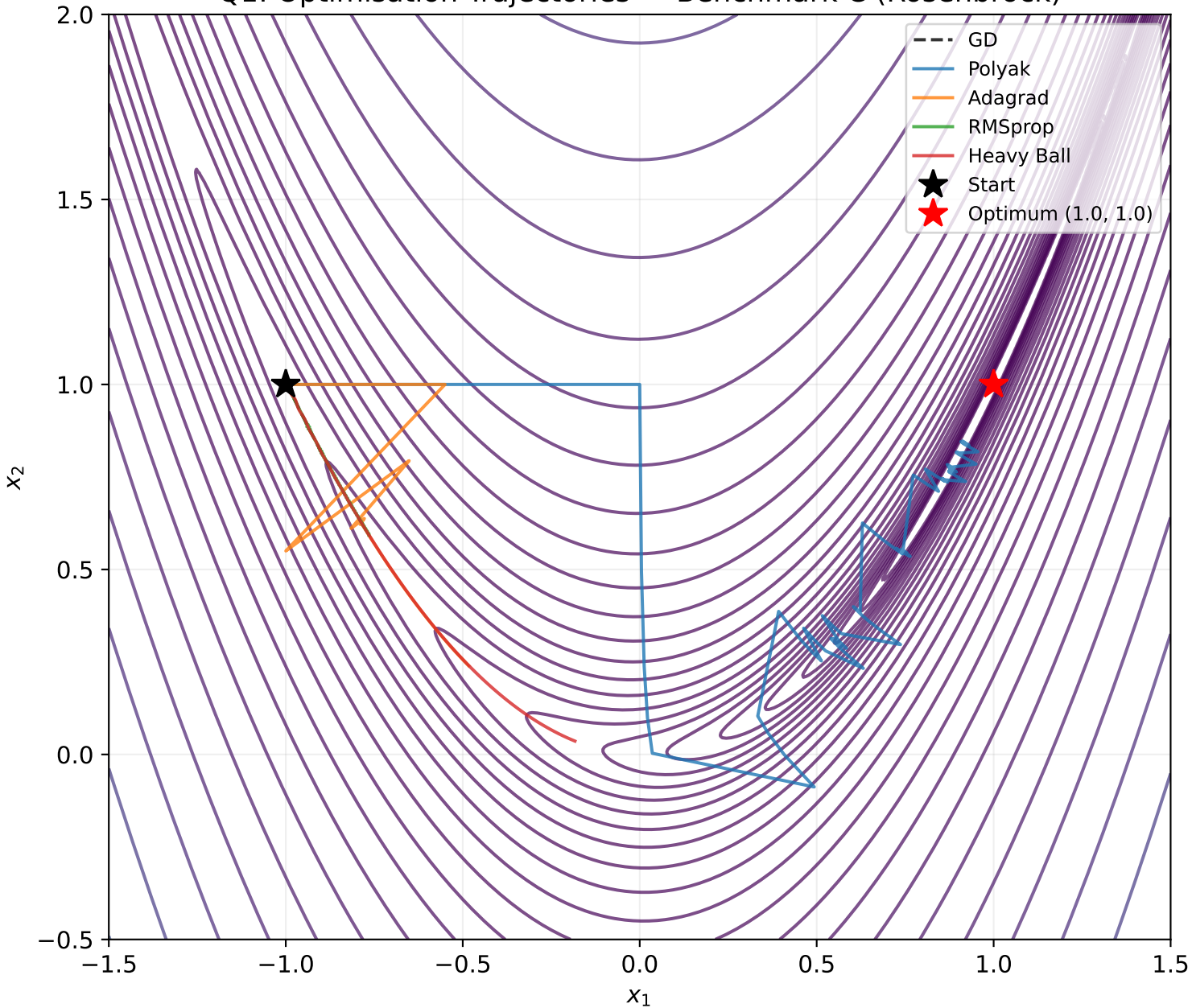
Q1: Optimisation Trajectories — Benchmark C (Rosenbrock)
