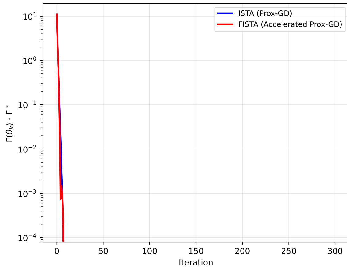
ISTA vs FISTA for LASSO ( \lambda = 0.2 , d = 10 )
