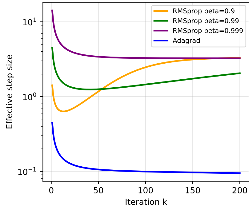
Adagrad vs RMSprop: Step Decay
