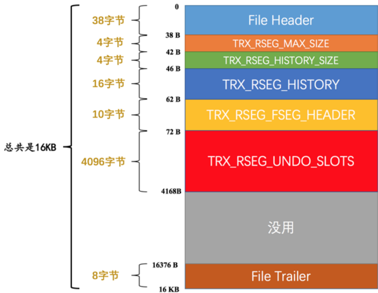
Rollback Segment Header结构示意图
