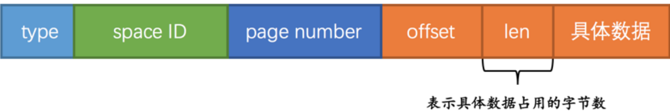
MLOG_WRITE_STRING类型的redo日志结构
