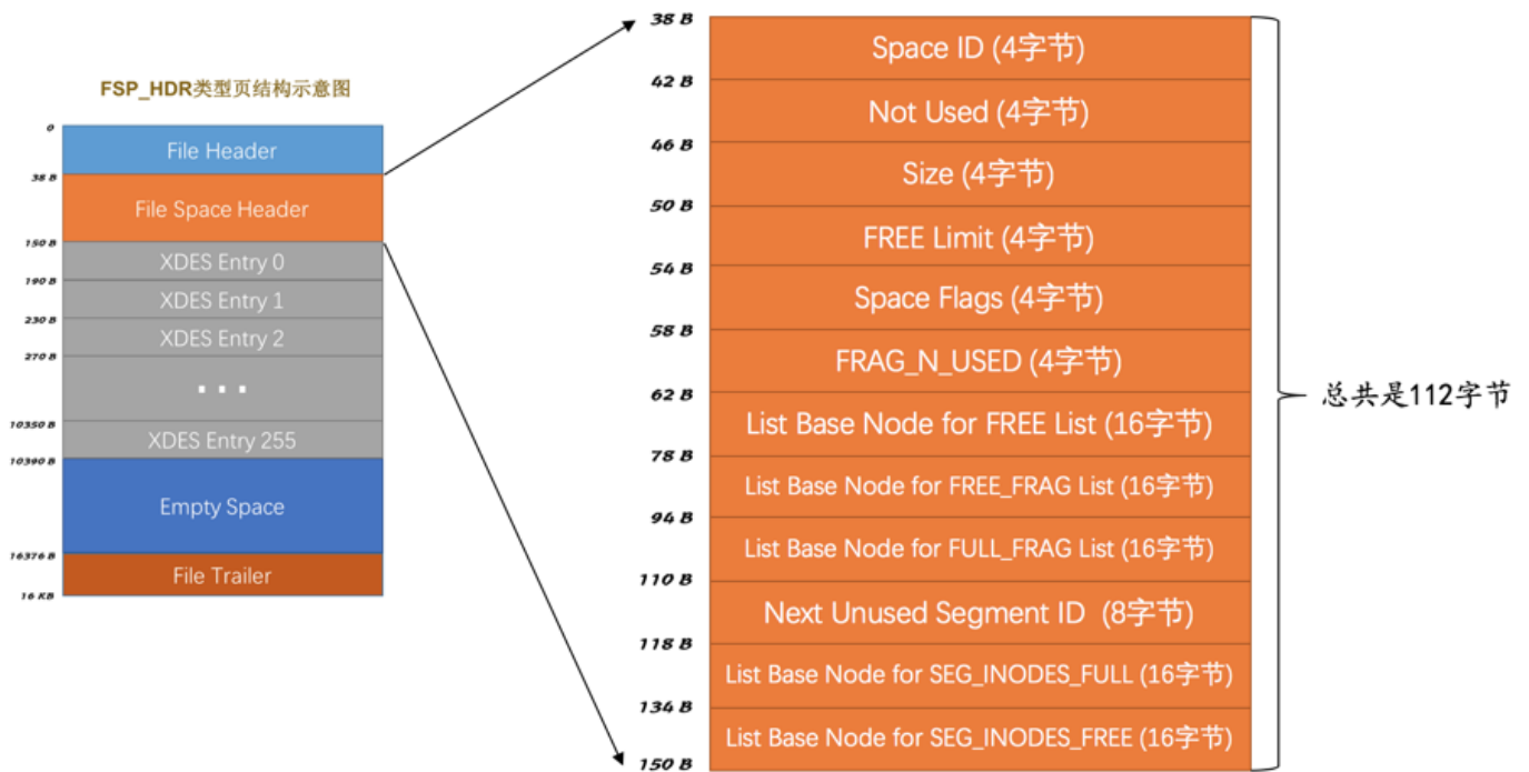
File Space Header结构示意图
