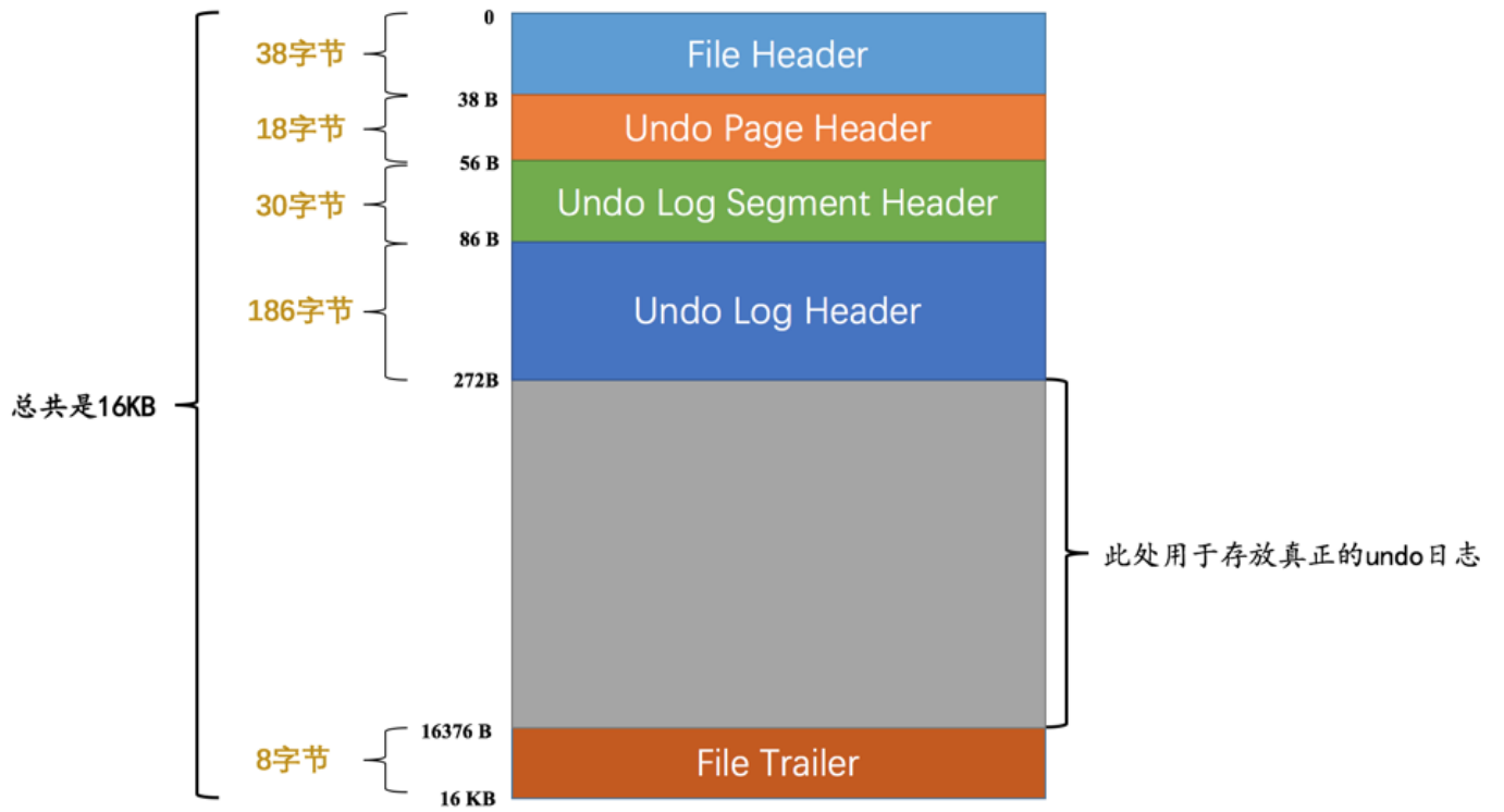
first undo page结构示意图
