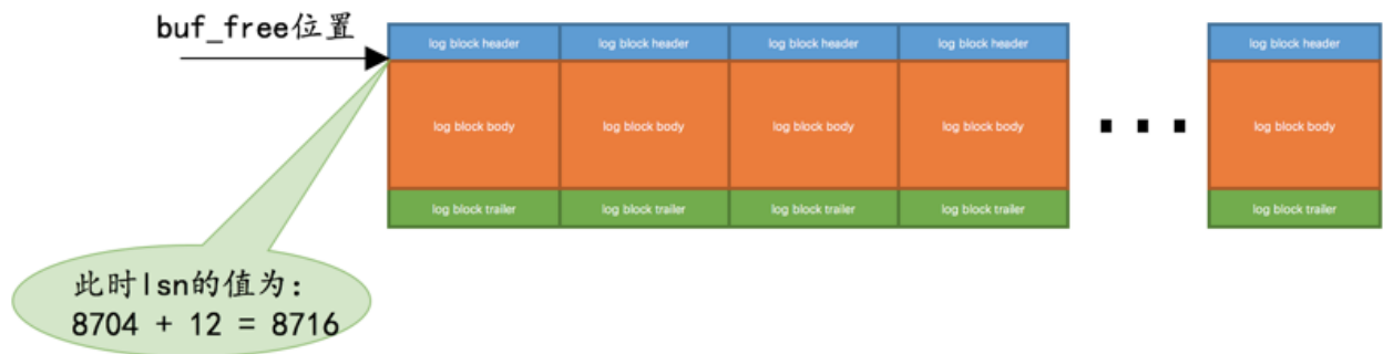
log buffer结构示意图
