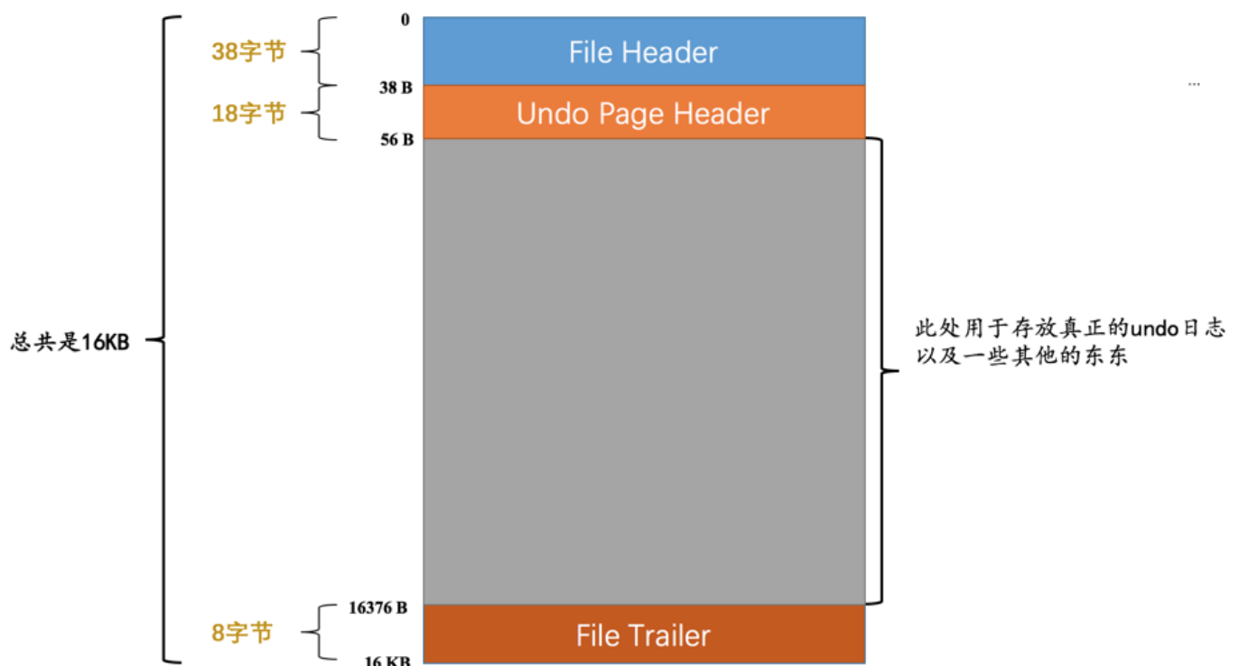
FIL_PAGE_UNDO_LOG页通用结构示意图
