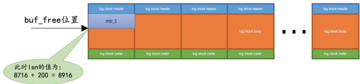
log buffer结构示意图
