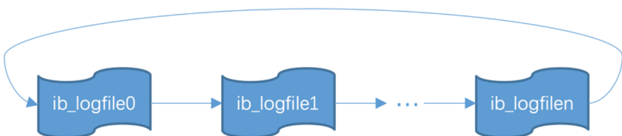
redo日志文件组示意图
