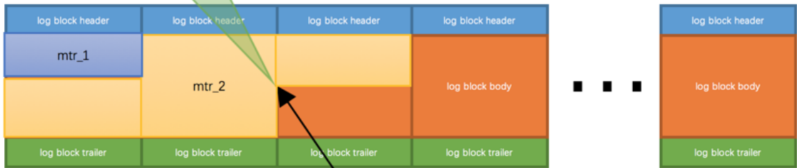
log buffer结构示意图
