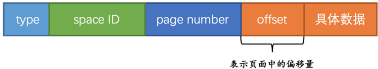
MLOG_8BYTE类型的redo日志结构
