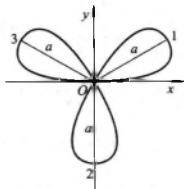
(16) 三叶玫瑰线
