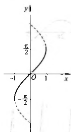
y = \arcsin x
