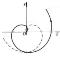
(10) 阿基米德螺线
