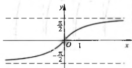
y = \arctan x
