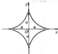
(7) 星形线(内摆线的一种)
