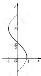
y = \arccos x
