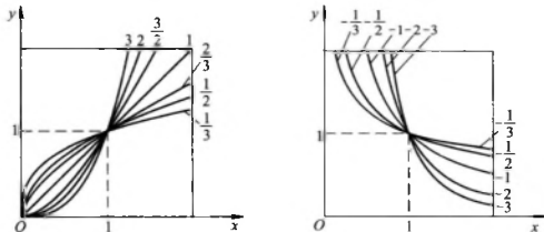
幂函数
