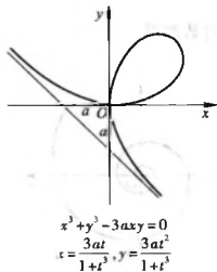
(6) 笛卡儿叶形线
