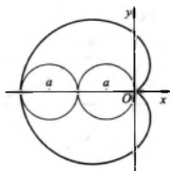
(9) 心形线(外摆线的一种)
