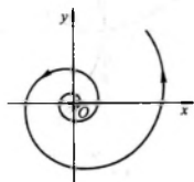
(11) 对数螺线
