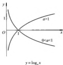
对数函数
