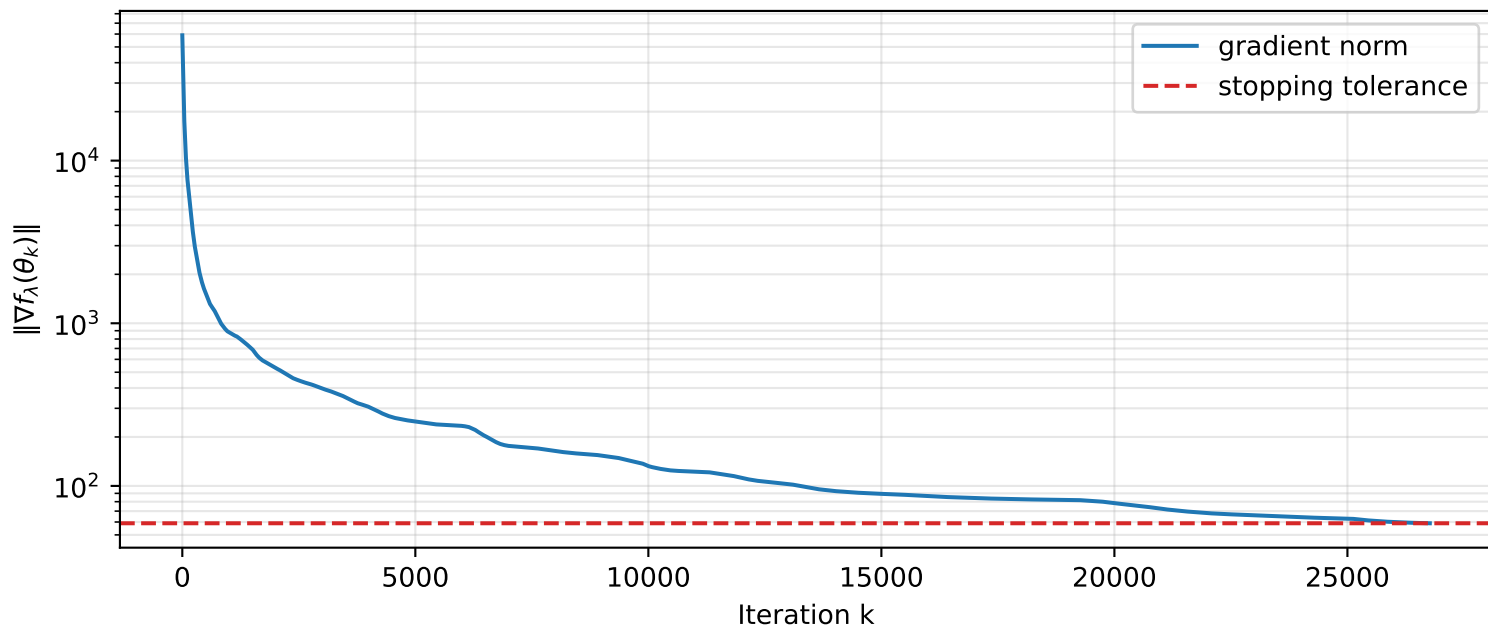
Gradient norm
