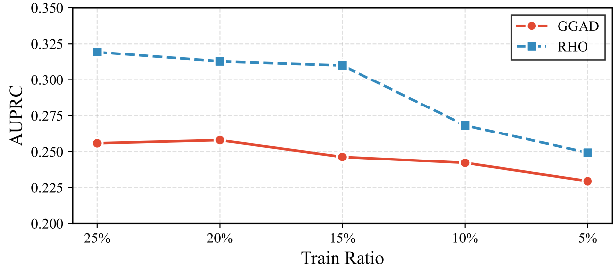
(b) AUPRC
