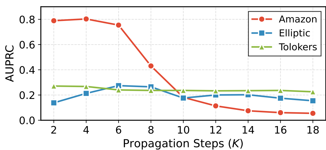
(b) AUPRC
