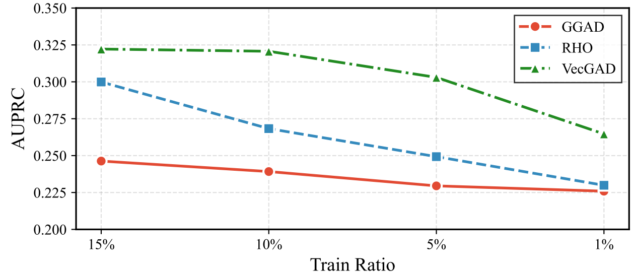
(b) AUPRC
