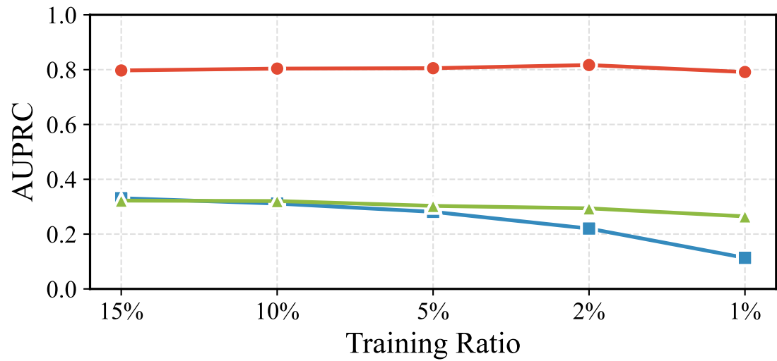
(b) AUPRC
