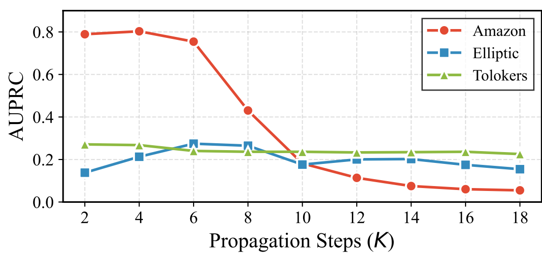
(b) AUPRC
