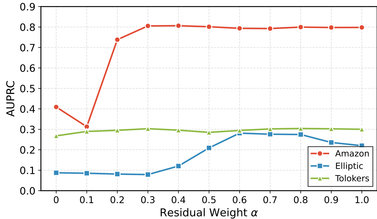
(b) AUPRC
