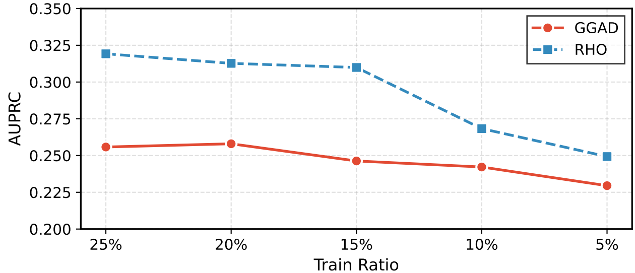
(b) AUPRC
