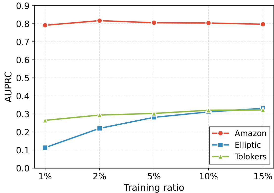
(b) AUPRC
