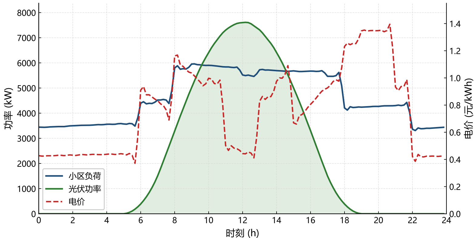
典型日负荷、光伏与电价曲线
