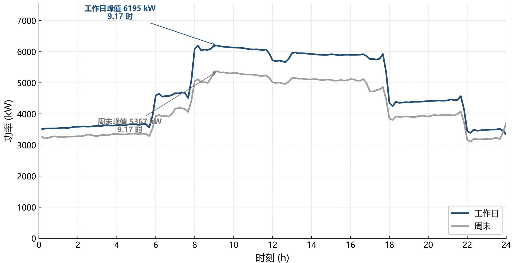
小区负载：工作日与周末平均日曲线
